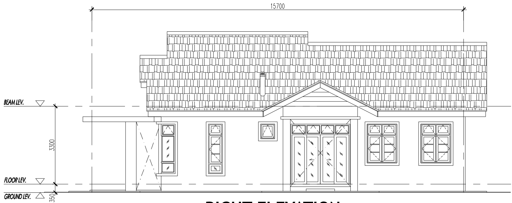
RIGHT ELEVATION
