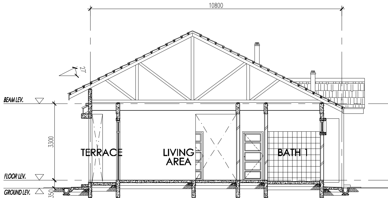
SECTION A-A
