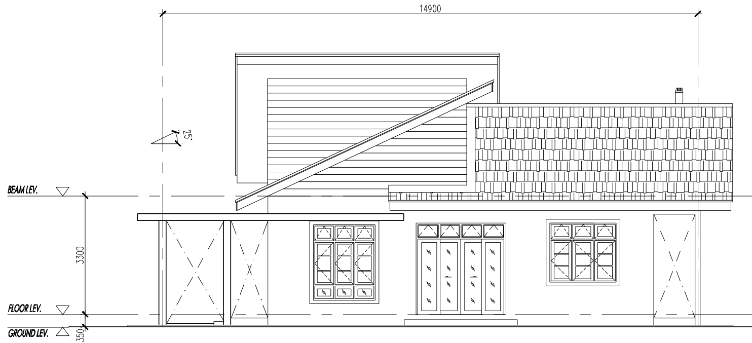
RIGHT ELEVATION
